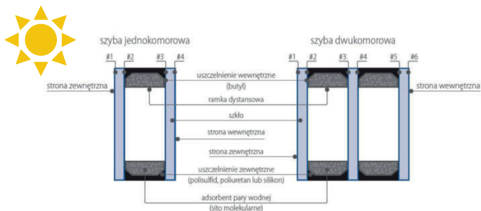
Rys. 1. Budowa szyby jednokomorowej i dwukomorowej z oznaczeniem części składowych i pozycji szkła
